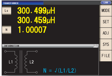
트랜스 측정 모드 권수비 측정 (Information) 화면
