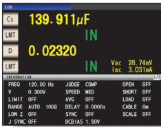
LCR 모드 DC 바이어스 설정 시
